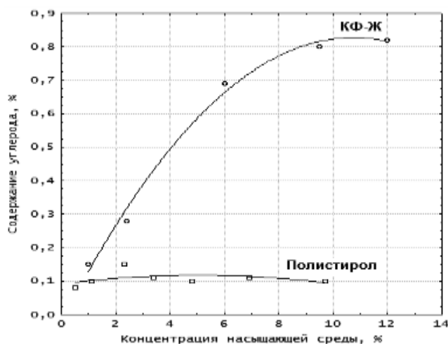
Рис. 2. Влияние концентрации растворов полимеров на содержание углерода в износостойком слое
