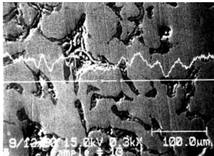
Рис. 5. Распределение углерода и микроструктура износостойкого слоя
