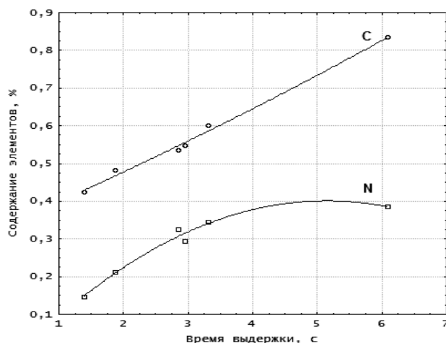
Рис. 4. Влияние времени выдержки при температуре напекания на содержание углерода и азота в износостойком слое ( T = 950^{\circ}\text{C} )
