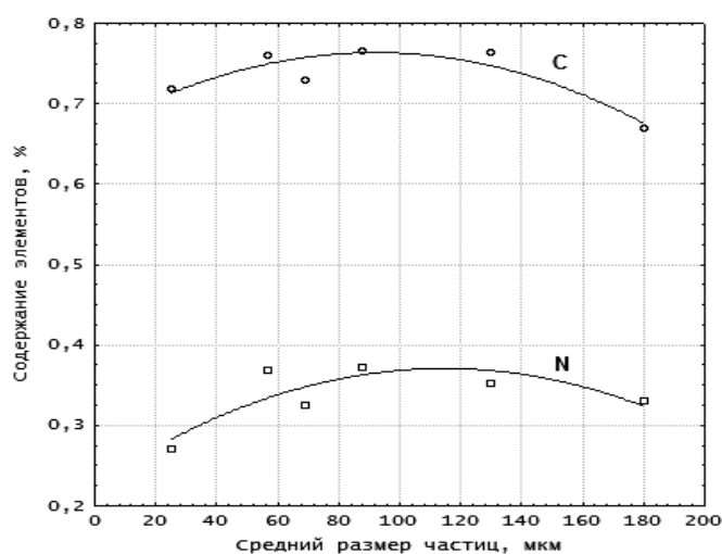
Рис. 3. Влияние размера частиц металлического порошка, модифицированного смолой КФ-Ж, на содержание углерода и азота в износостойком слое
