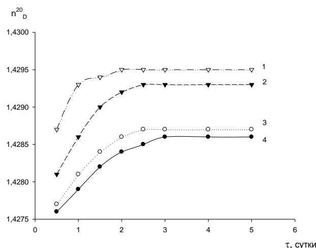
Рис. 1. Кинетические кривые адсорбции олигомера КФ-Ж из водного раствора на поверхности частиц различных фракций порошка ПЖВ: 1 - 25 мкм, 2 - 50 мкм, 3 - 90 мкм, 4 - 130 мкм
